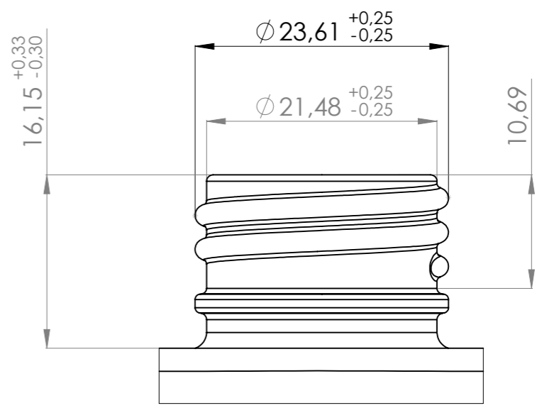
DETTAGLIO B SCALA 2 : 1
