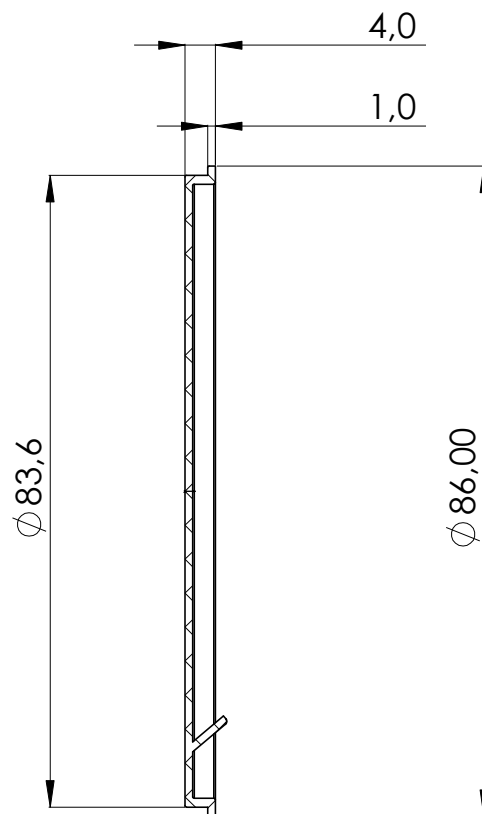
SEZIONE E-E
