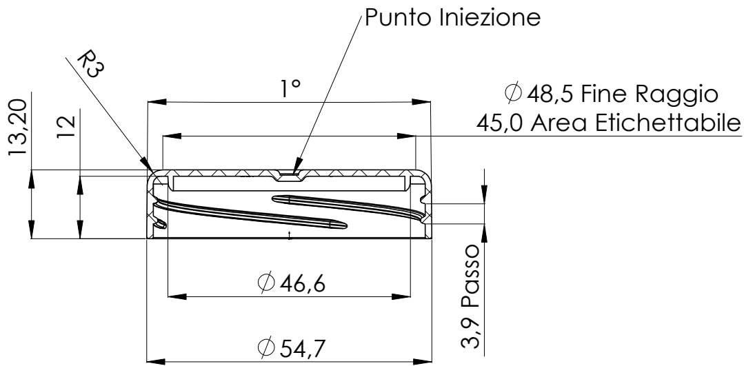
SEZIONE E-E
