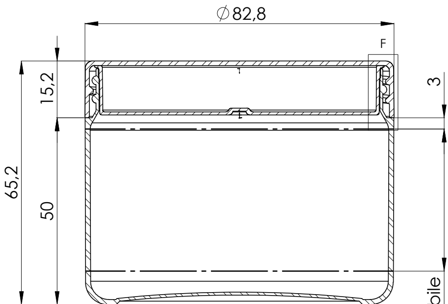
SEZIONE E-E
