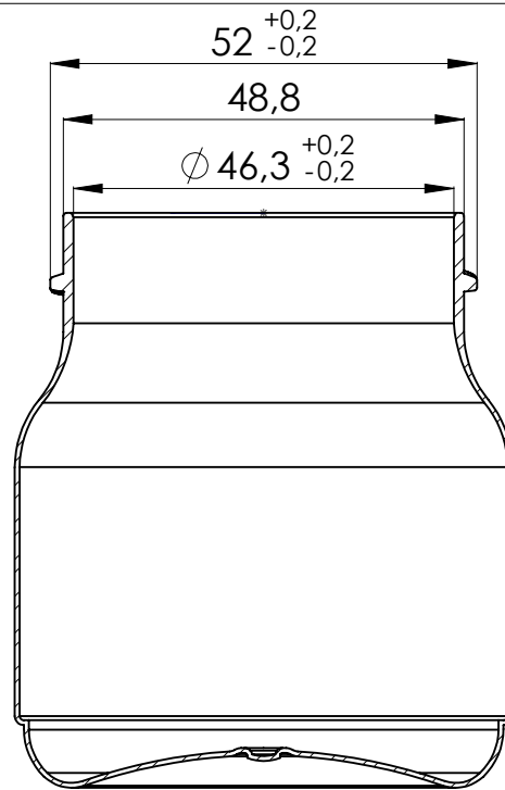
SEZIONE A-A
