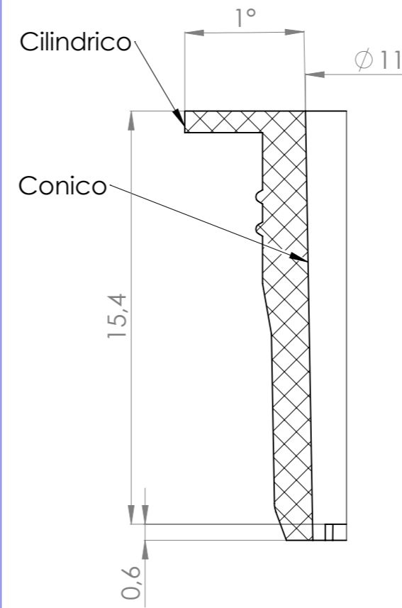
DETTAGLIO K SCALA 5 : 1
